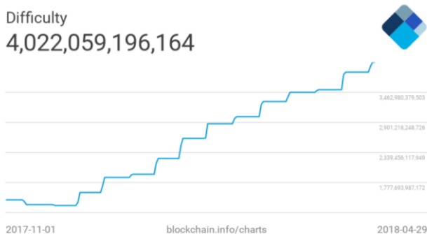
图 2.3: 比特币挖矿难度变化图
