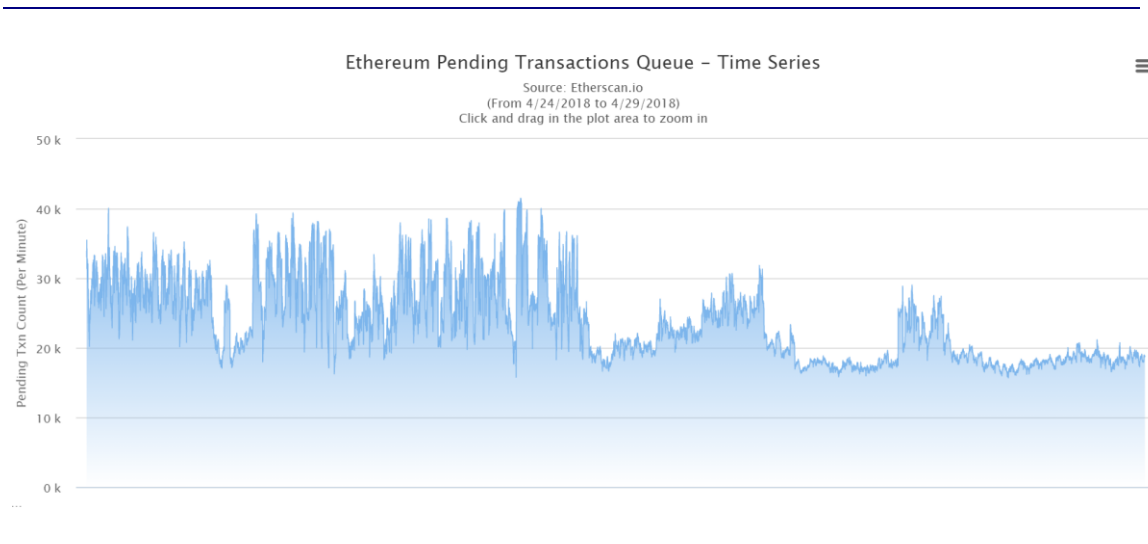
图 2.12：以太坊未确认交易数图
